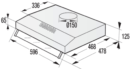
Hotte d'aspiration norme EURO / 60 cm WHU 629 AX/M
